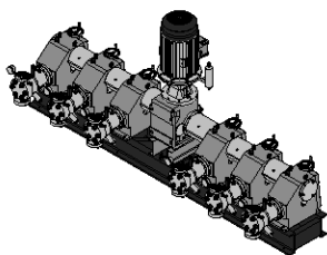
P_ORL_057_SW1 Bomba múltiple Orlita® MF6S 1400/50
