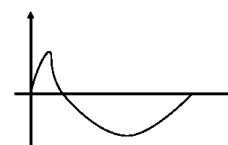
P_SI_0104_SW Esquema 3: carrera de impulsión corta, carrera de aspiración larga
