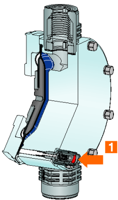
P_SI_0065_C1 1: Indicación de rotura de la membrana
