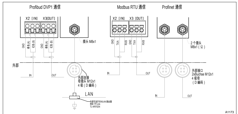
插图 1: 通讯模块的端子图
