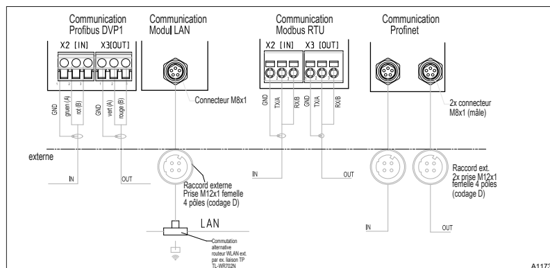
Fig. 1 : Plan de connexion des modules de communication
