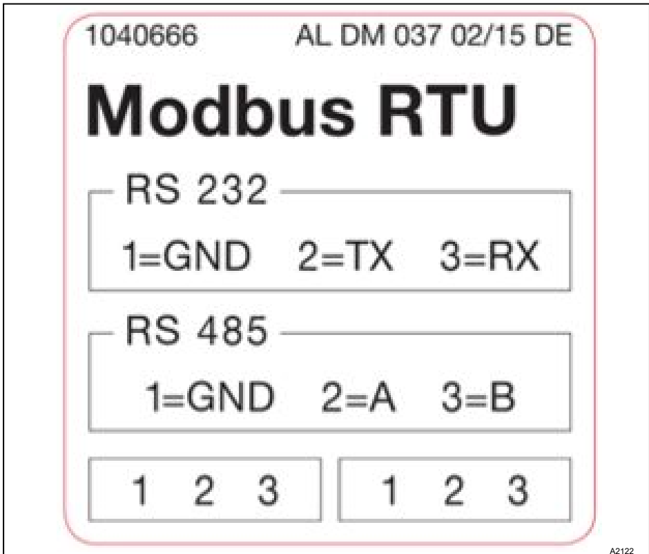
Abb. 1: Modbus-Anschlussklemmen
